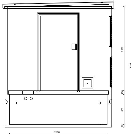
Voorraanzicht
