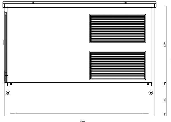
Zijaanzicht Rechts
